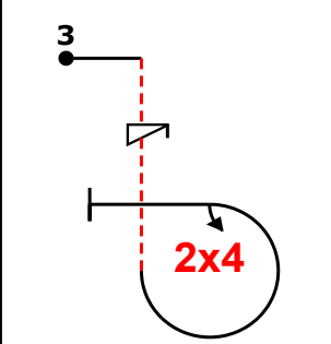
Fig C 8.6.4.3(13) 9.11.1.4(5) 9.4.3.2(5) K: 23
